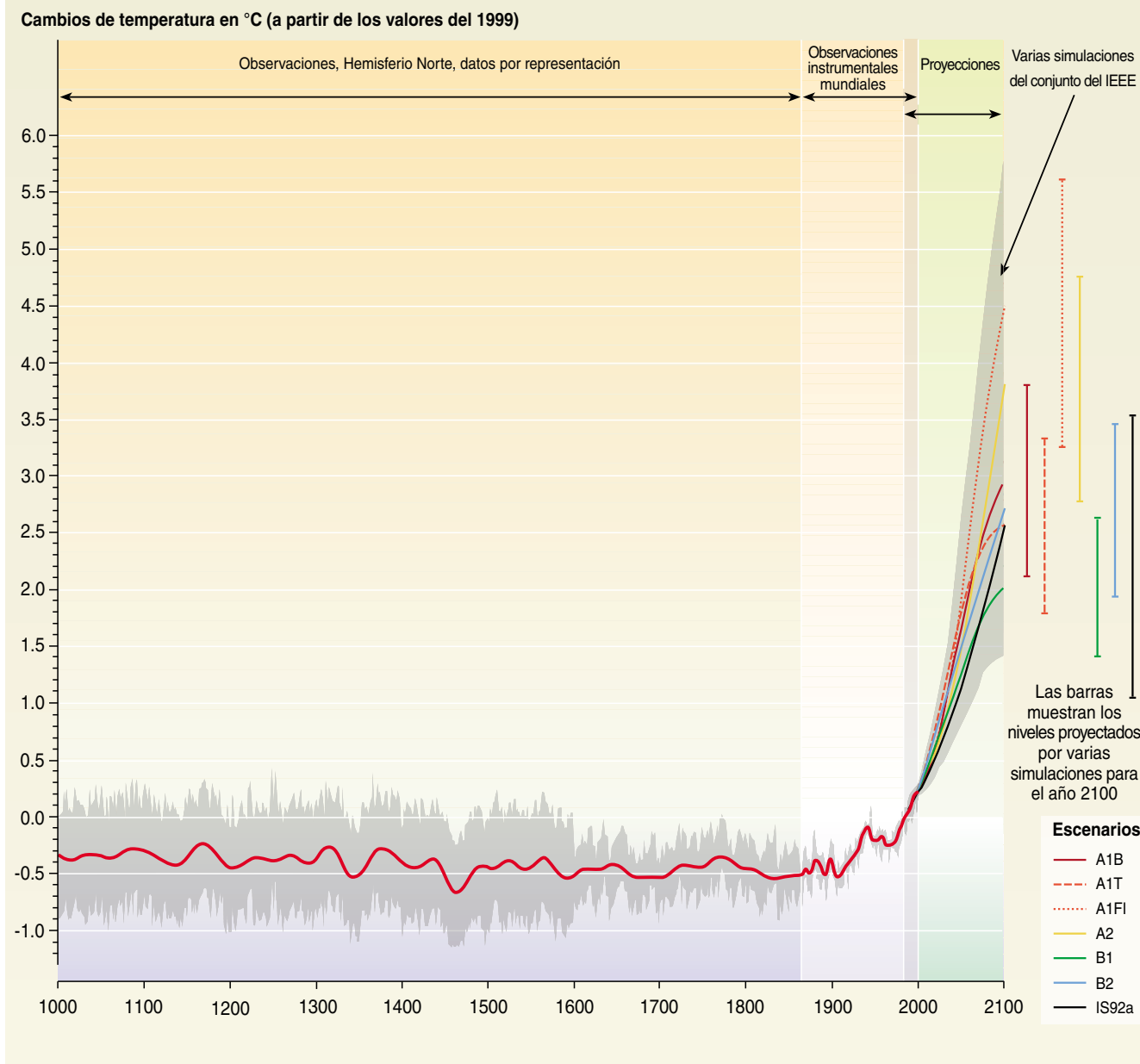
Figura RRP-10b: Se muestran las variaciones en la temperatura media de la superficie en el Hemisferio Norte durante el periodo 1000–1860 (no se dispone de los datos correspondientes para el Hemisferio Sur) extraídos a partir de datos por representación (anillos de los árboles, corales, testigos de hielo y registros históricos). La línea muestra una media en 50 años, el área gris, el límite de confianza del 95 por ciento en los datos anuales. Para el periodo 1860–2000 se muestran las observaciones de variaciones anuales y mundiales de la temperatura media de la superficie obtenidas del registro instrumental. La línea muestra la media por decenios. Para el periodo 2000–2100, se muestran las proyecciones de la temperatura media mundial de la superficie para los seis escenarios ilustrativos del IEEE y los del IS92a, estimadas mediante una simulación con sensibilidad climática media. El área gris marcada 'Varias simulaciones del conjunto del IEEE' muestra la gama de resultados de los 35 escenarios del IEEE además de aquellos obtenidos de una gama de simulaciones con diferentes sensibilidades climáticas. La escala de temperaturas se determina a partir del valor para 1990; la escala es diferente de la utilizada en la Figura RRP-2.
