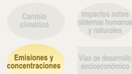
(f) Concentraciones de CO 2 (ppm)
